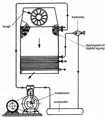
63. ábra. Hűtőkörfolyamat (nagyított légűtő-egységgel)
