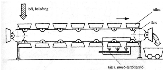
61. ábra. Vizsgáló tálcás szalag
