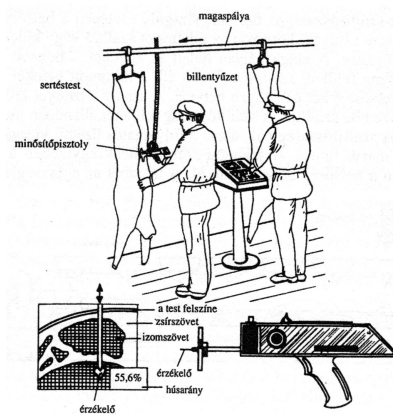
62. ábra. Henessy sertésminősítő berendezés
