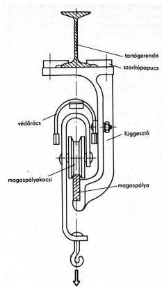
10. ábra. A magaspálya-szerkezet metszete
