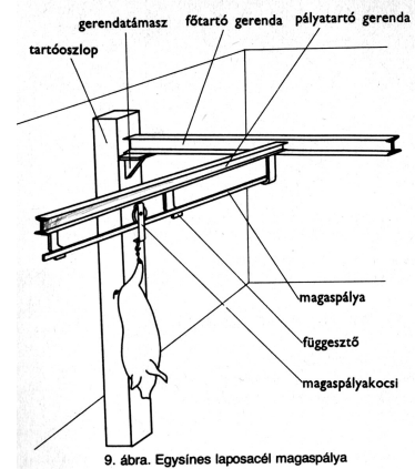
9. ábra. Egysínes laposacél magaspálya
