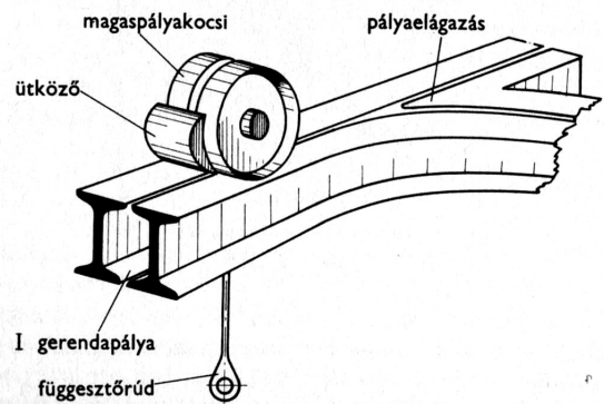
13. ábra. Kétsínes magaspálya
