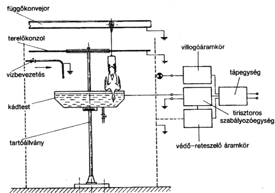
79. ábra. Folyadékös elektromos baronfikábító berendezés
