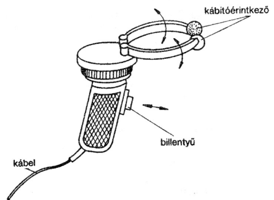
78. ábra. Baronfikábító fogó
