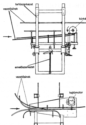
91. ábra. Meyn baronfióló gép
