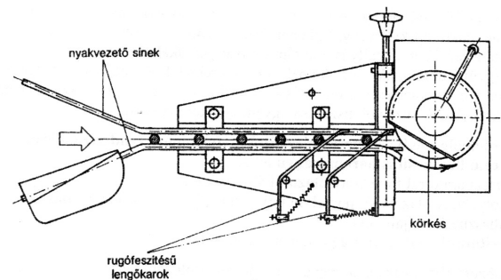
90. ábra. Stork baronfióló gép
