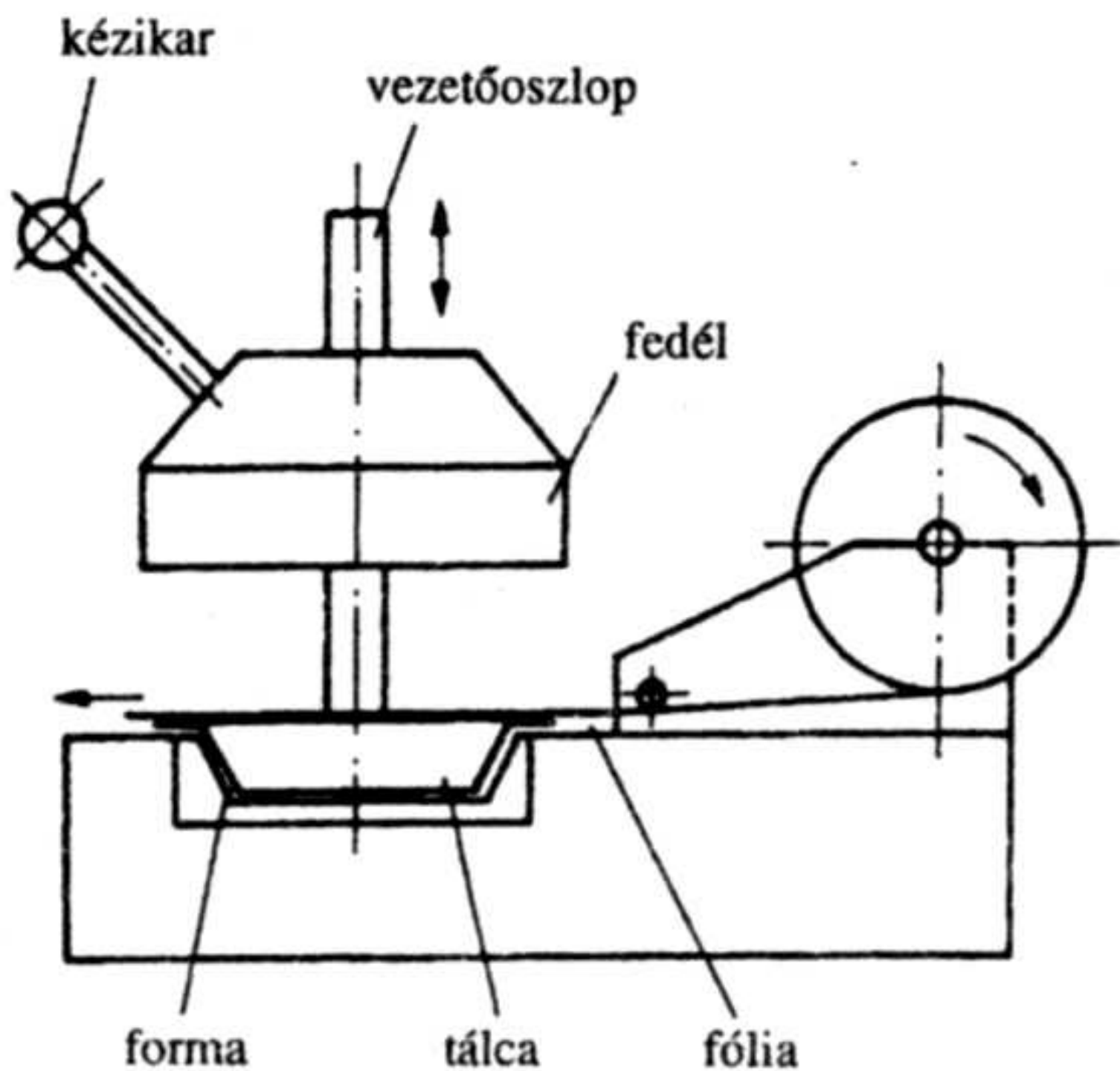
182. ábra. Kézi tálcás csomagológép
