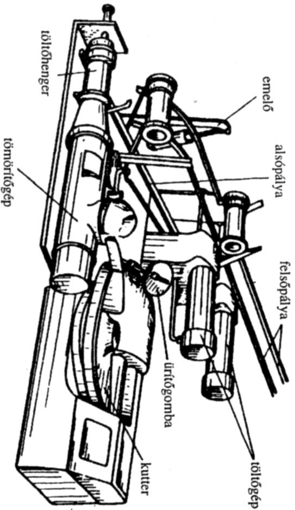
154. ábra. Szalámi gyártó gépsor
