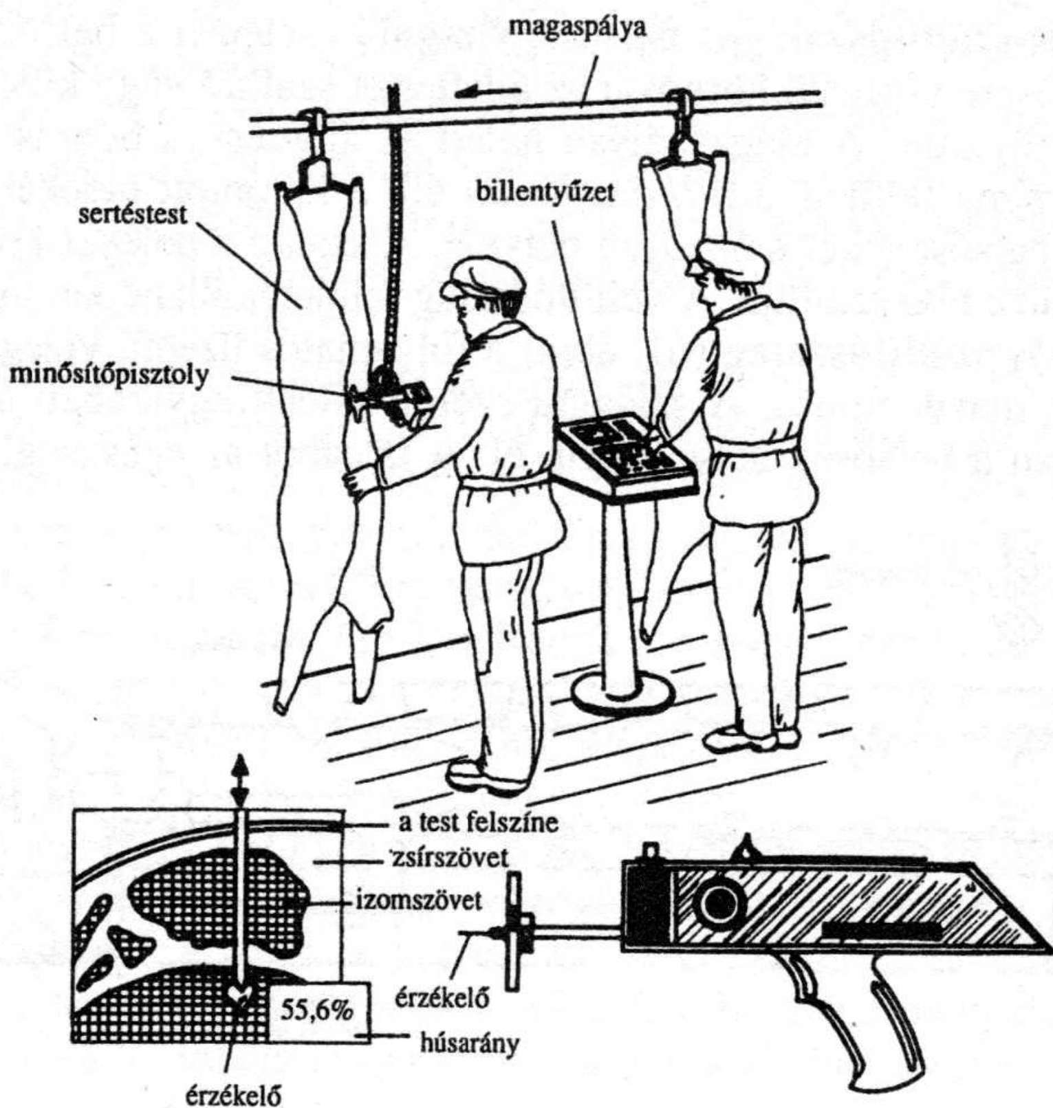
62. ábra. Henessy sertésminősítő berendezés
