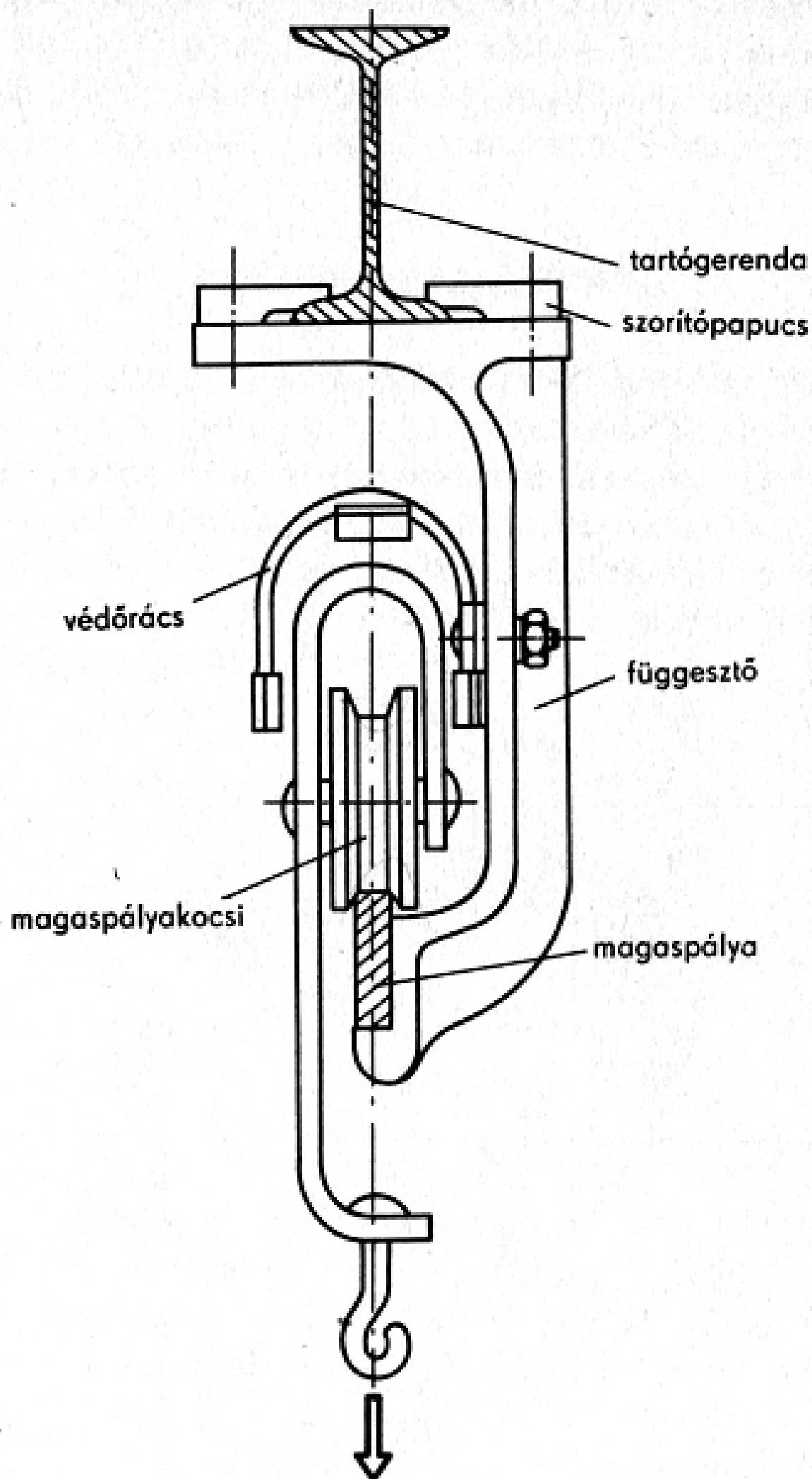
10. ábra. A magaspálya-szerkezet metszete
